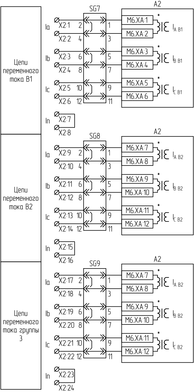
Цепи переменного тока
