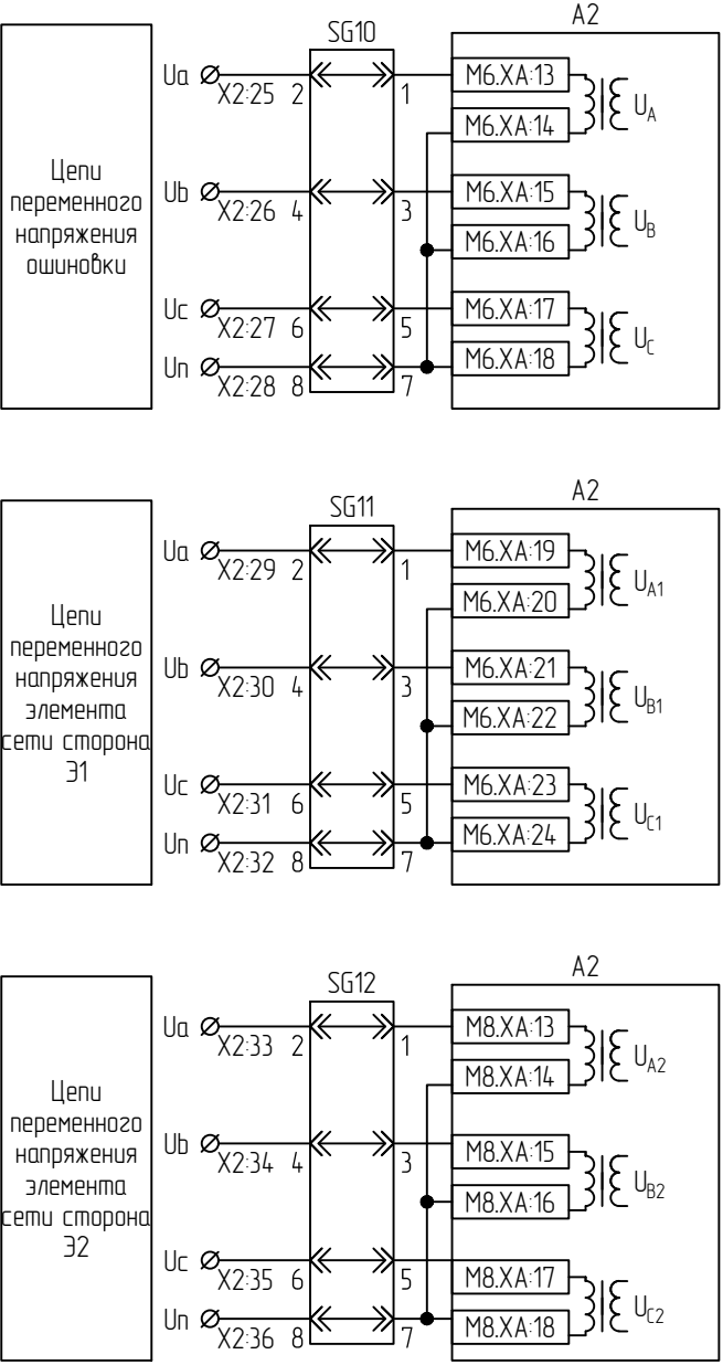
Цепи переменного напряжения
